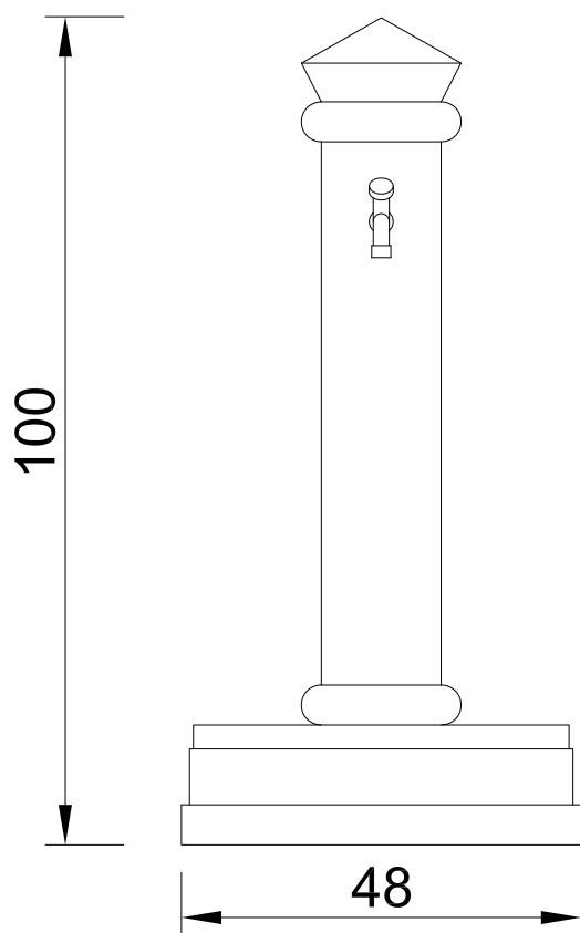
PROSPETTO FRONTALE
