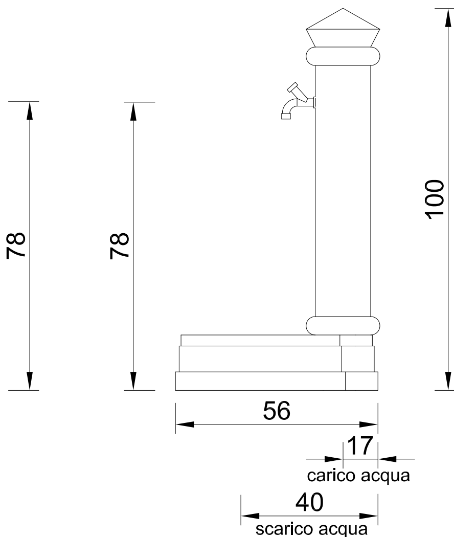
PROSPETTO LATERALE
